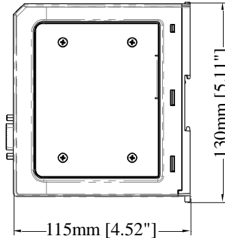
侧视图
